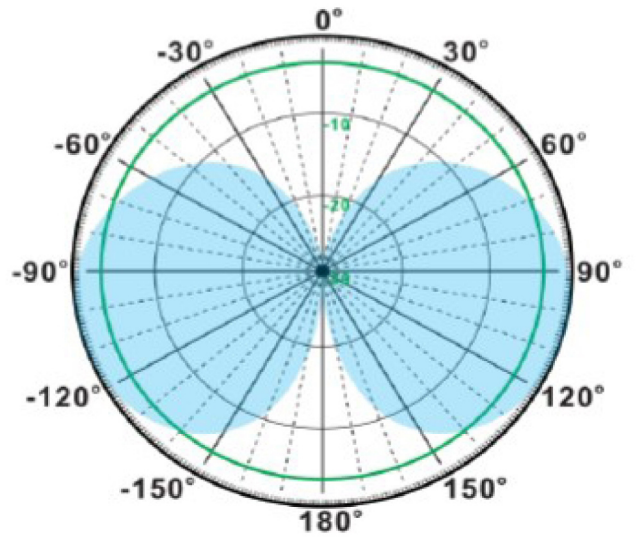
V-Plane
