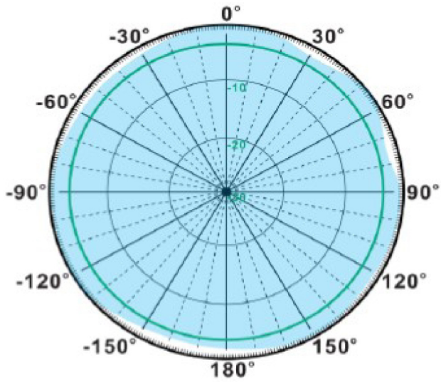
H-Plane
