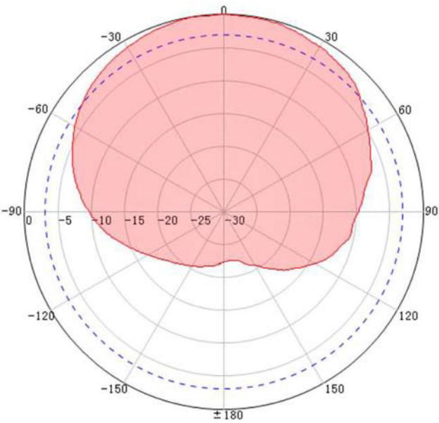
700MHz V Plane
